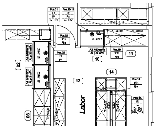
Ausschnitt Einrichtungsplan mit Installationsangaben
