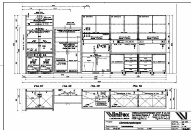
Ausführungszeichnung (Wandabwicklung)
