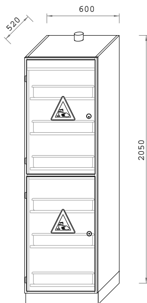
zweitürig zur getrennten Lagerung von Säuren und Laugen
