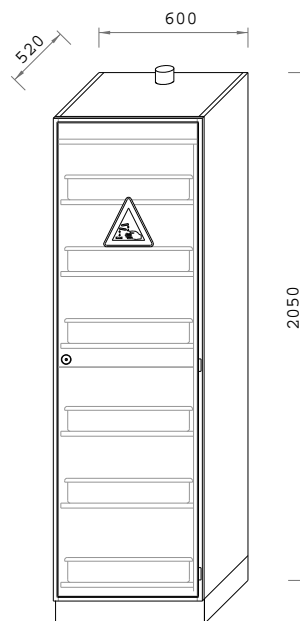
eintürig für Säuren oder Laugen
